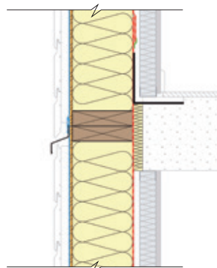
Coupe verticale sur FOB filante
