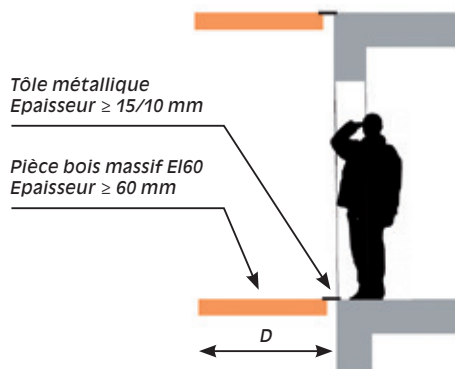
Schéma de principe d'un dispositif pouvant participer au C+D, selon l'IT249
