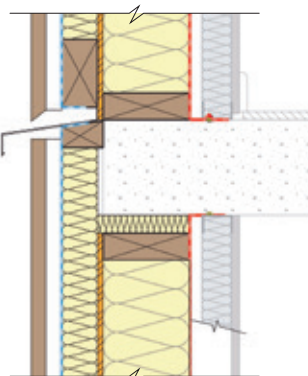
Coupe verticale sur FOB interrompue
