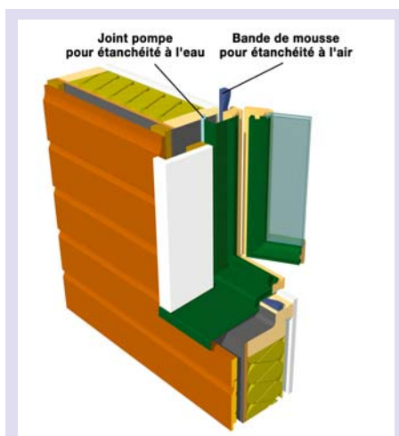
Exemple de soin particulier à apporter au calfeutrement en périphérie des châssis de menuiseries.
