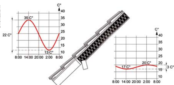
Conception d'une toiture pour une réduction d'amplitude de facteur 10 et un déphasage de 12 heures
