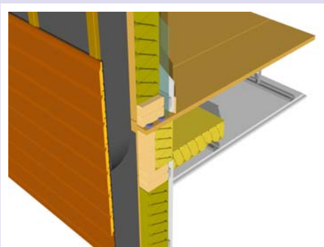
Exemple de joint de mousse comprimée en pied de doublage ou entre lisses pour que l'air ne puisse pas s'infiltrer aux liaisons planchers/panneaux de façade et se diffuser sous les plinthes.
