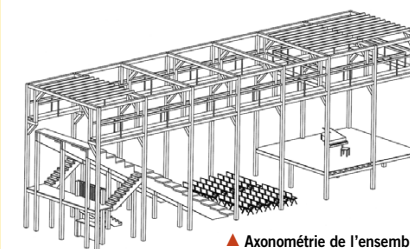
▲ Axonométrie de l'ensemble de la structure.
